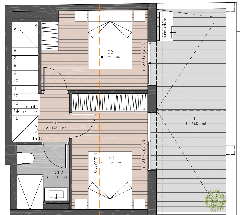
PLANTA SOTACOBERTA
