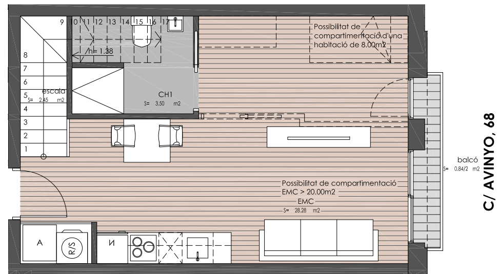
PLANTA TERCERA
