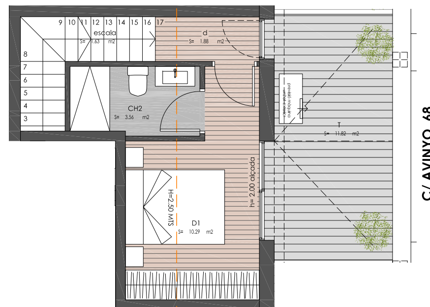
PLANTA SOTACOBERTA
