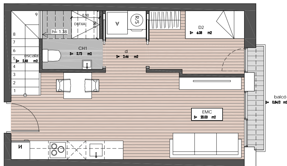
PLANTA TERCERA
