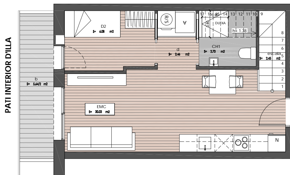
PLANTA TERCERA
